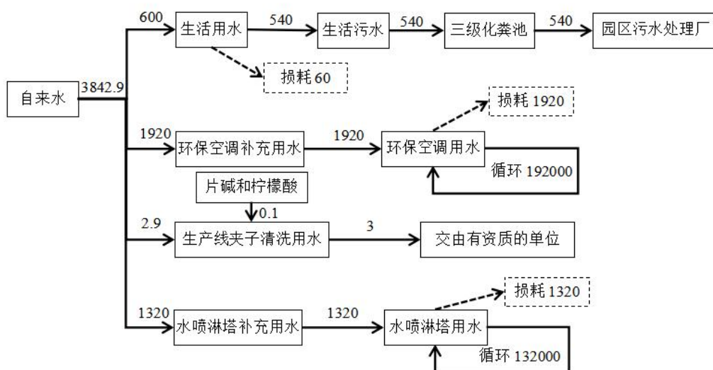
图 1 项目水平衡图（单位： \text{m}^3/\text{a} ）
