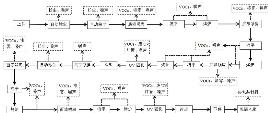
图2 项目自动真空镀膜生产工艺流程图
