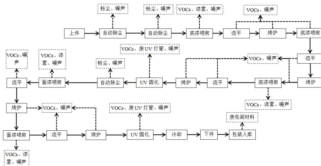
图3 项目自动喷涂生产工艺流程图
