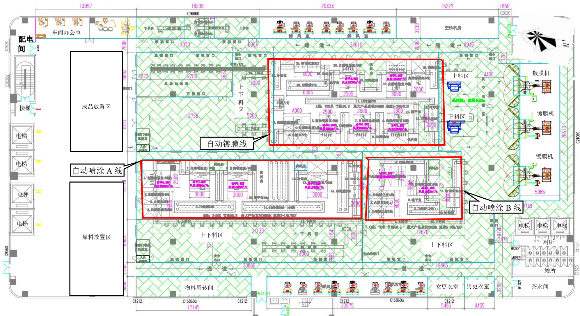
附图 5-2 项目车间平面布置图（10 楼）
