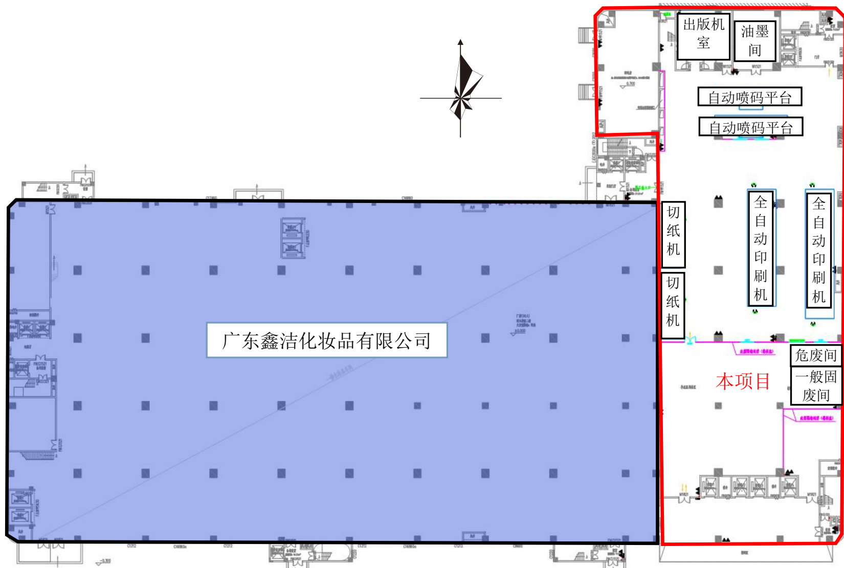
附图 4-1 项目 1 楼车间平面布置图
